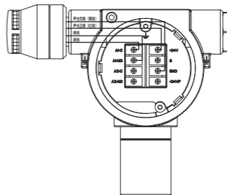
D610/D650/D630接线图
