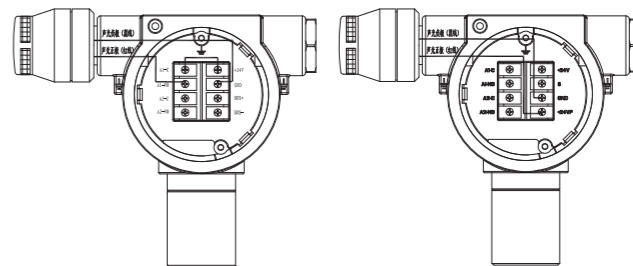
D630接线图
